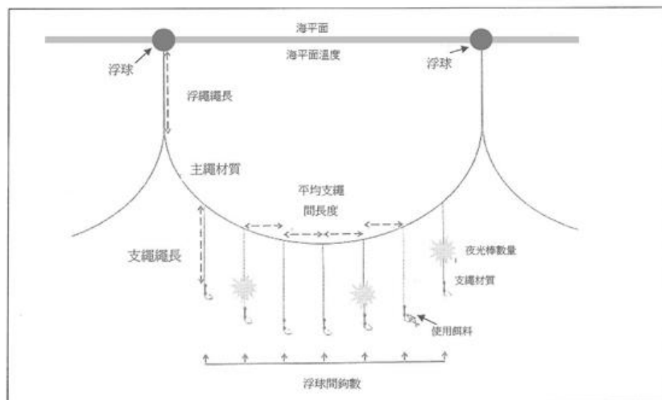
投繩作業時漁具設置之示意圖
