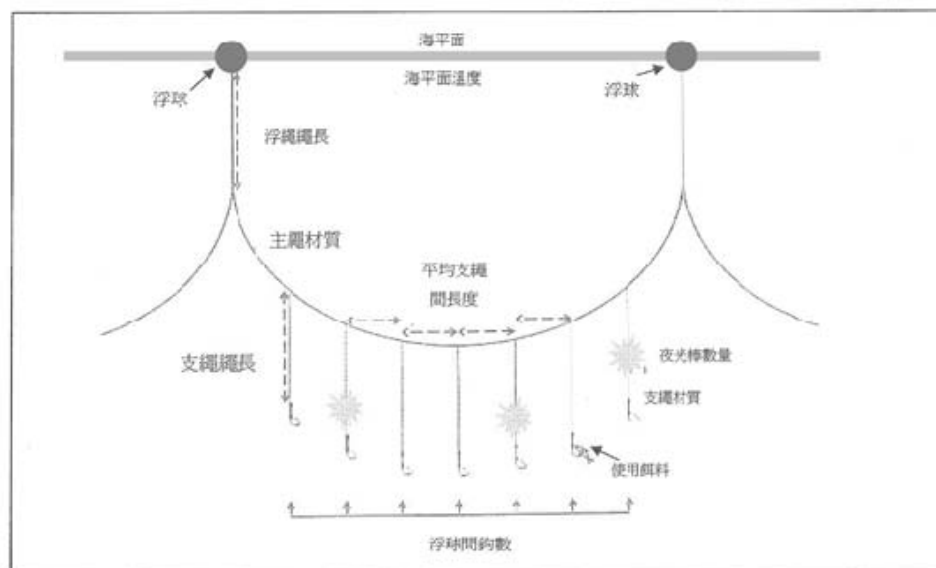
投繩作業時漁具設置之示意圖
